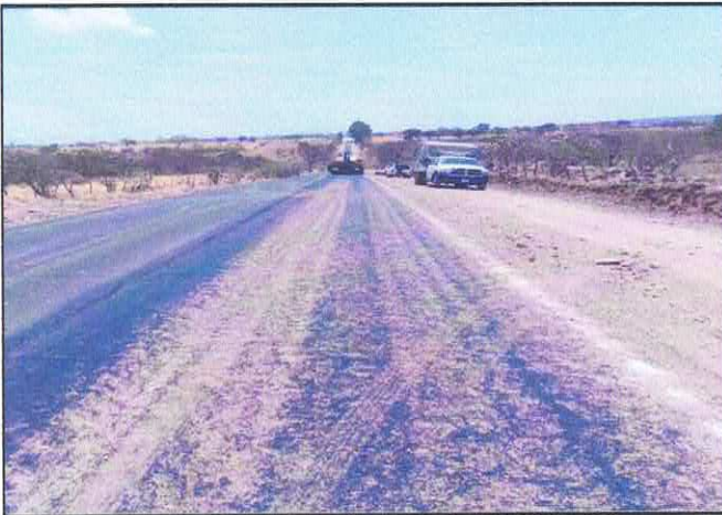
TENDIDO Y COMPACTACIÓN DE CARPETA ASFALTICA.
